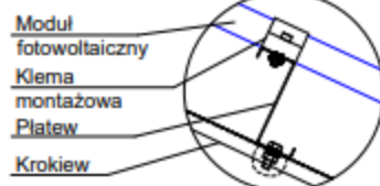
DETAL A
