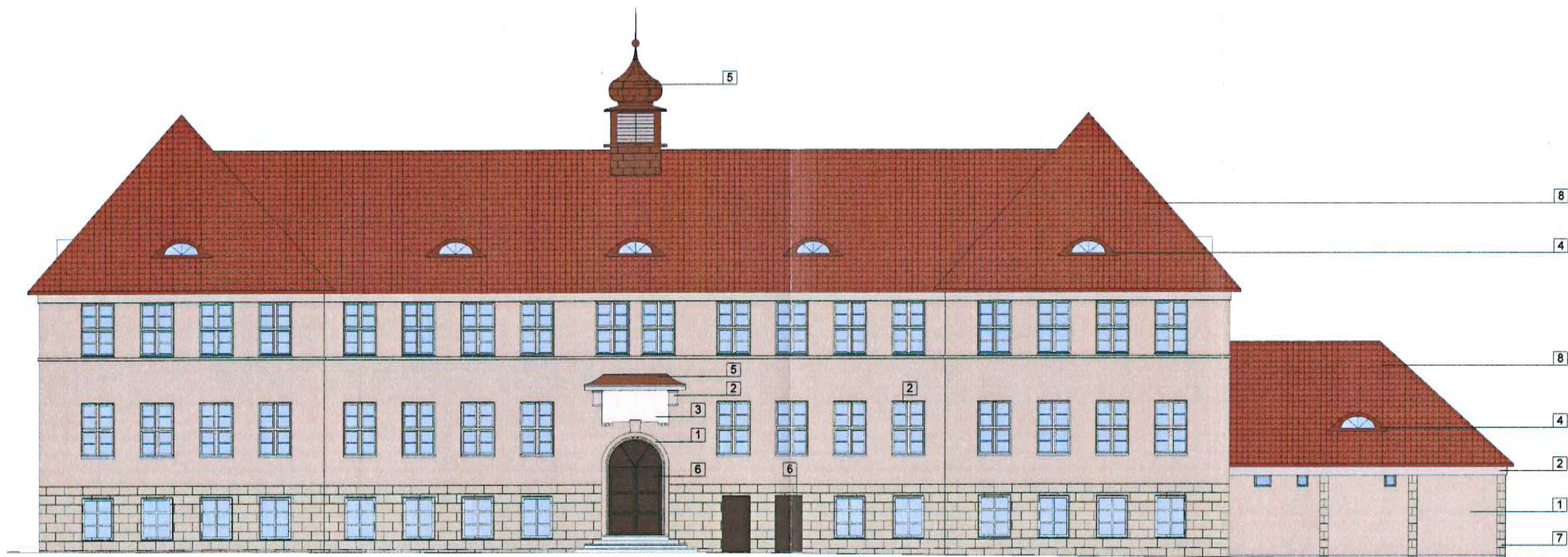
ELEWACJA POLUDNIOWO - ZACHODNIA
